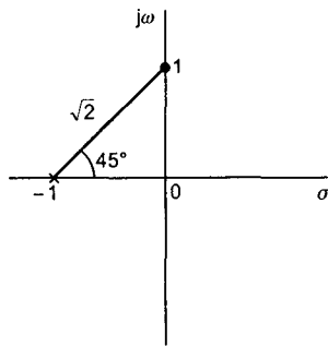
Figura 11.2 G(j\omega)
