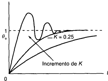
Figura 9.8 Respuesta del sistema de la figura 9.6 a una entrada escalón unitario
