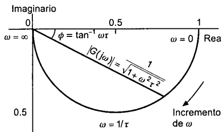
Figura 11.20 Trazado de Nyquist para G(s) = 1/(1 + \tau s)
