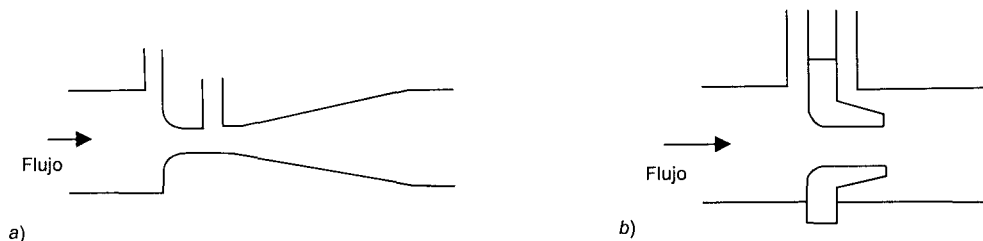
Figura 12.14 Medidores de flujo de boquilla: a) boquilla Venturi, b) boquilla de flujo
