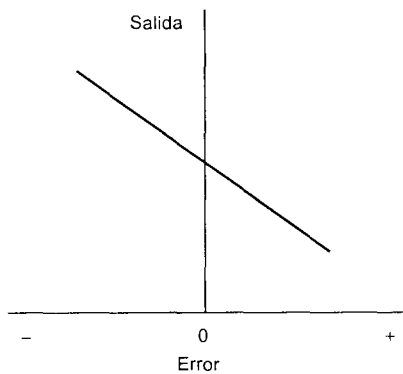
Figura 1.20 Control proporcional
