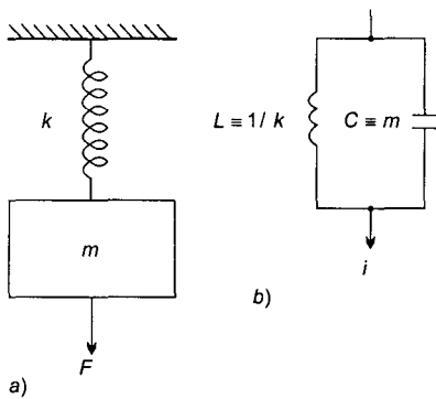
Figura 2.20 Analogías mecánica y eléctrica
