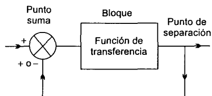
Figura 6.1 Elementos de un diagrama de bloques
