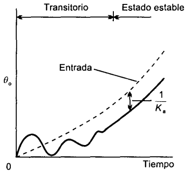
Figura 7.8 Error en estado estable con entrada parabólica
