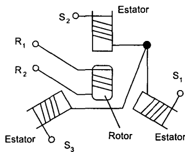
Figura 12.10 Elemento sincro
