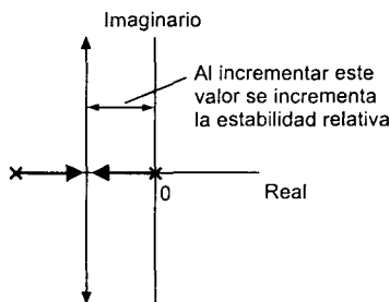
Figura 9.27 Estabilidad relativa
