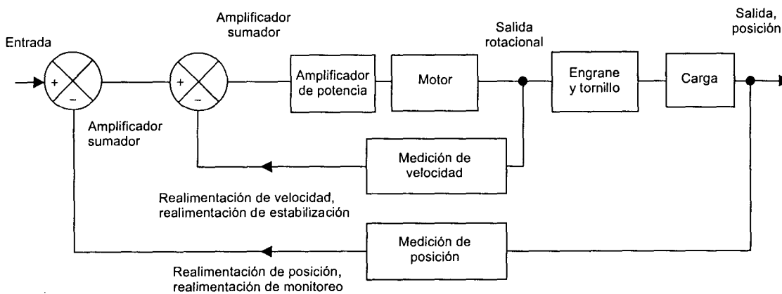
Figura 12.31 Sistema con realimentación de velocidad
