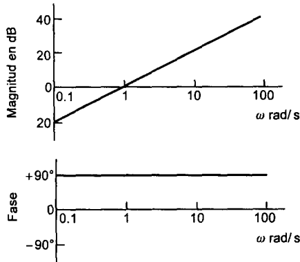
Figura 11.7 Trazas de Bode para un cero en el origen
