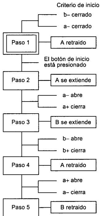
Figura 13.7 Diagrama de funciones
