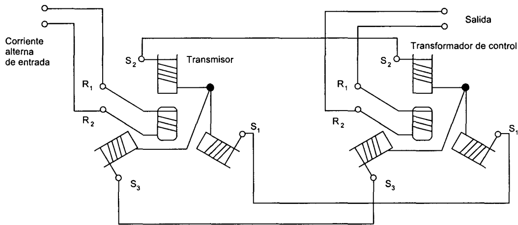
Figura 12.11 Detector de error con sincros
