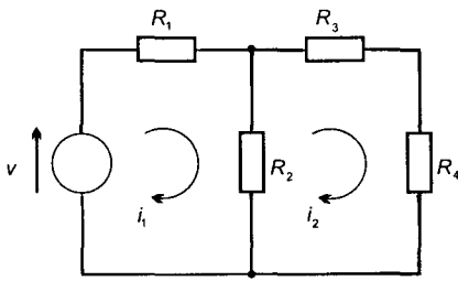
Figura 2.11 Circuito para ilustrar el análisis de mallas
