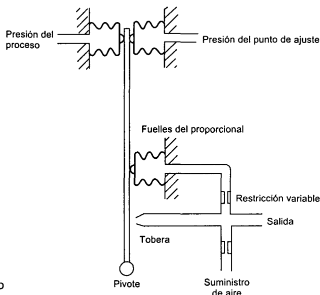
Figura 10.32 Controlador PD neumático
