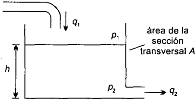
Figura 2.26 Capacitancia hidráulica
