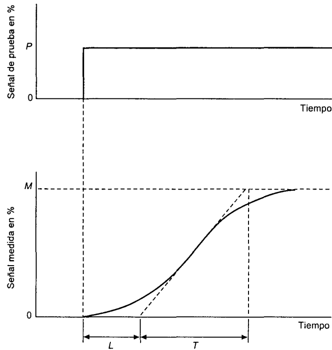
Figura 10.16 Curva de reacción de proceso
