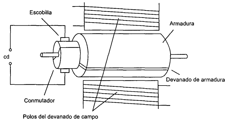
Figura 12.17 Elementos básicos de un motor de cd
