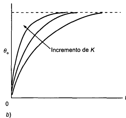
Figura 9.4 Respuesta del sistema de la figura 9.2 a: a) una entrada impulso, b) una entrada escalón
