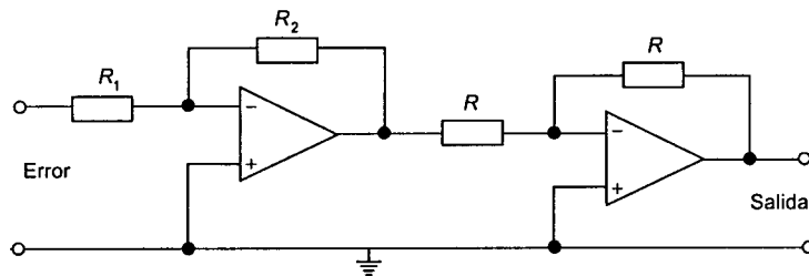
Figura 10.24 Controlador proporcional
