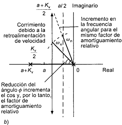
Figura 10.19 El efecto de la realimentación de velocidad: a) sin, b) con realimentación de velocidad
