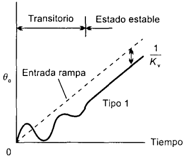
Figura 7.7 Error en estado estable con entrada rampa
