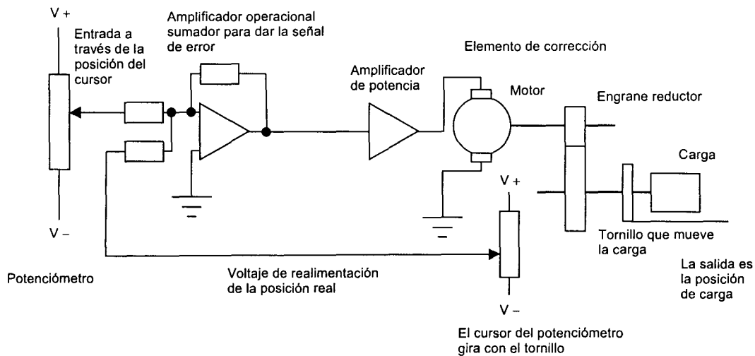
Figura 12.28 Sistema de control de posición
