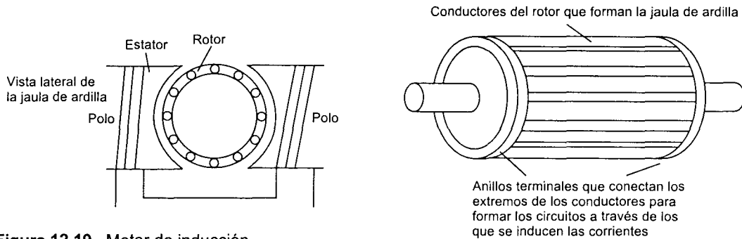
Figura 12.19 Motor de inducción
