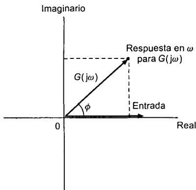
Figura 11.19 Trazado de un punto sobre un diagrama de Nyquist
