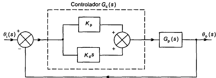
Figura 10.12 Control proporcional derivativo
