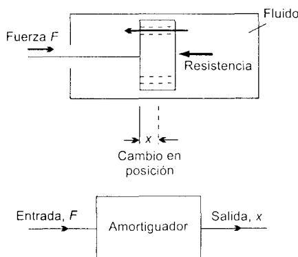
Figura 2.2 Un bloque funcional mecánico: el amortiguador
