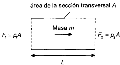
Figura 2.27 Inertancia hidráulica
