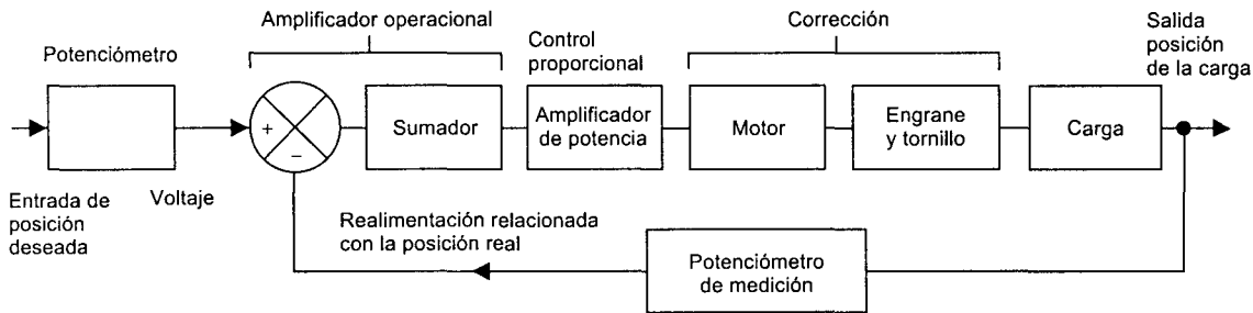
Figura 12.29 Sistema de control de posición
