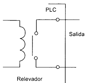
Figura 13.14 Canal de salida tipo relevador
