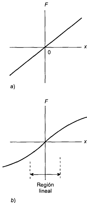
Figura 2.40 a) resorte ideal, b) resorte real
