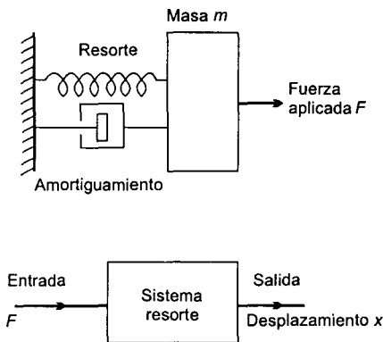
Figura 3.10 Un sistema resorte de segundo orden
