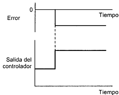
Figura 10.2 Sistema con control proporcional
