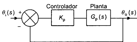
Figura 10.3 Sistema con control proporcional
