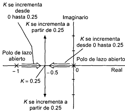
Figura 9.7 Lugares geométricos de las raíces para el sistema de la figura 9.6
