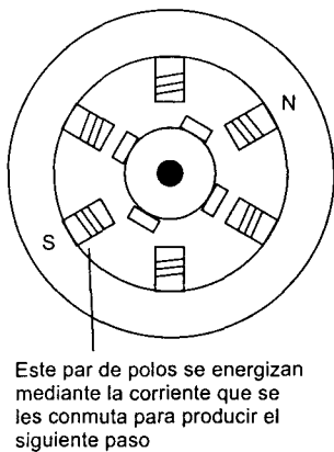
Figura 12.20 Motor de pasos de reluctancia variable
