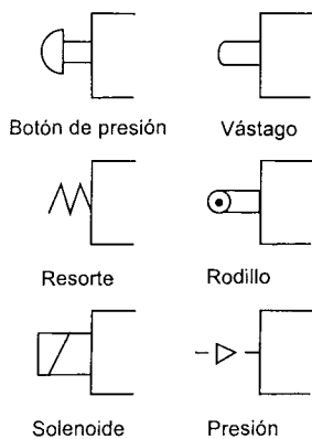
Figura 12.25 Actuadores para válvulas
