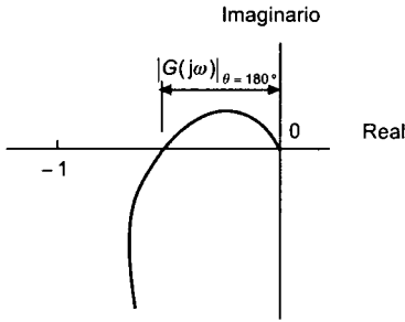
Figura 11.25 Margen de ganancia
