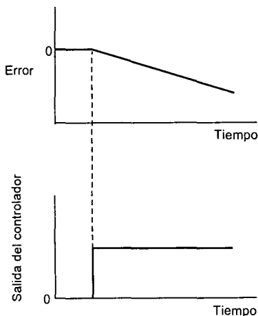
Figura 10.10 Control derivativo
