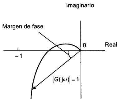
Figura 11.26 Margen de fase
