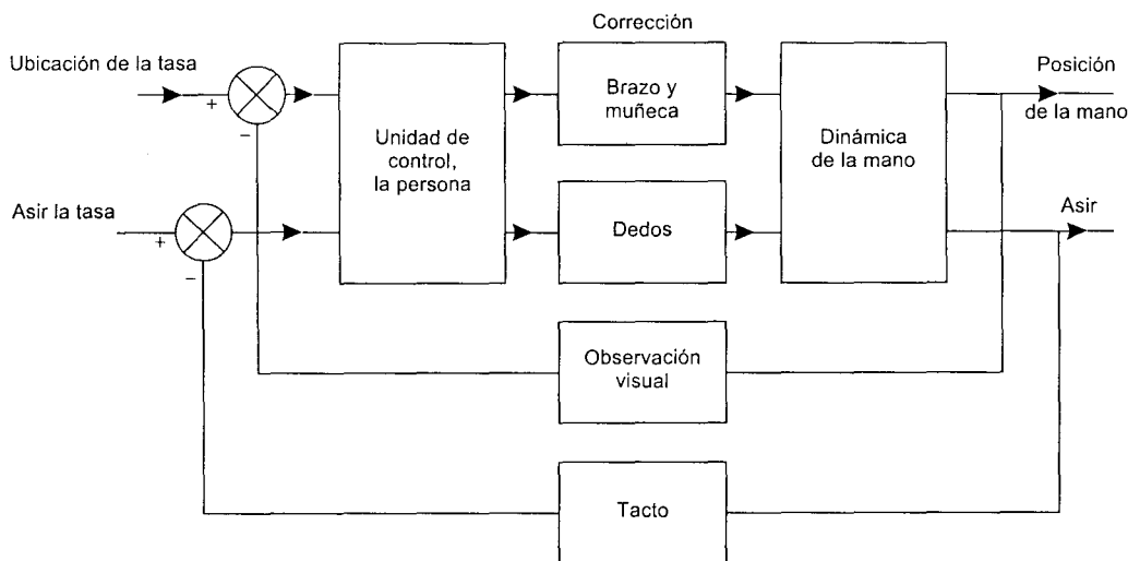
Figura 1.16 Levantar una tasa de café
