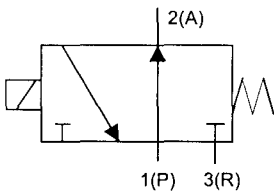
Figura 12.24 Símbolo de válvula
