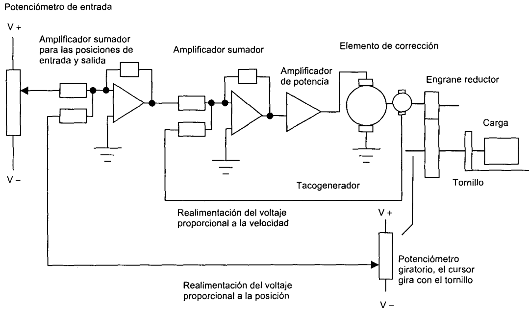
Figura 12.30 Sistema con realimentación de velocidad
