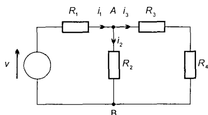
Figura 2.10 Circuito para ilustrar el análisis de nodos
