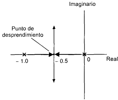
Figura 9.18 Punto de desprendimiento de G_o(s) = K/s(\sigma + 1)
