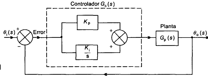
Figura 10.7 Control proporcional integral
