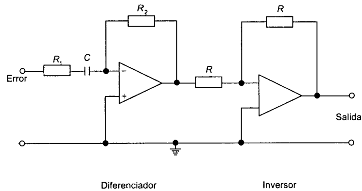
Figura 10.27 Controlador derivativo
