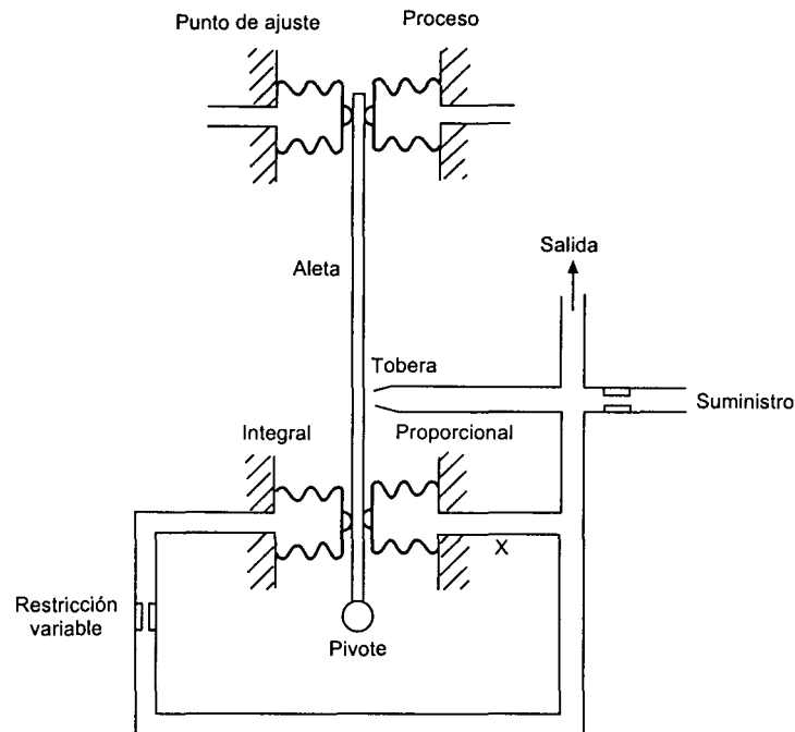
Figura 10.31 Controlador PI neumático
