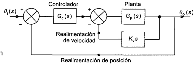
Figura 10.18 Sistema con realimentación de velocidad y posición
