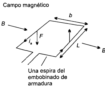
Figura 2.37 El motor de cd:
