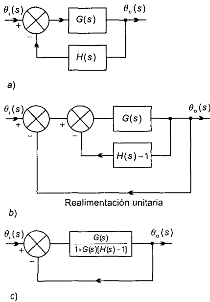
Figura 7.3 a) Sistema de control en lazo cerrado, b) conversión en realimentación unitaria, c) sistema equivalente con realimentación
