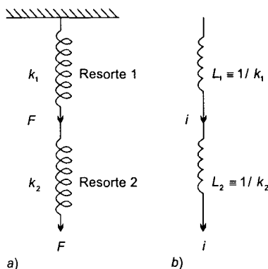
Figura 2.18 Analogías mecánica y eléctrica
