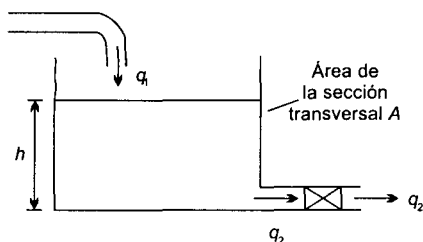
Figura 2.28 Un sistema hidráulico
