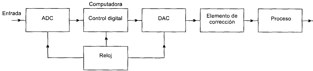
Figura 1.22 Sistema de control digital en lazo abierto para sistemas en tiempo continuo
