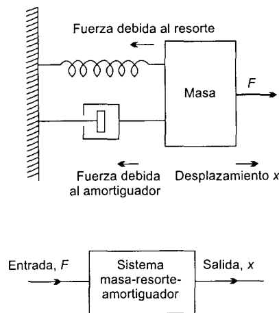
Figura 2.4 Sistema masa-resorte-amortiguador
