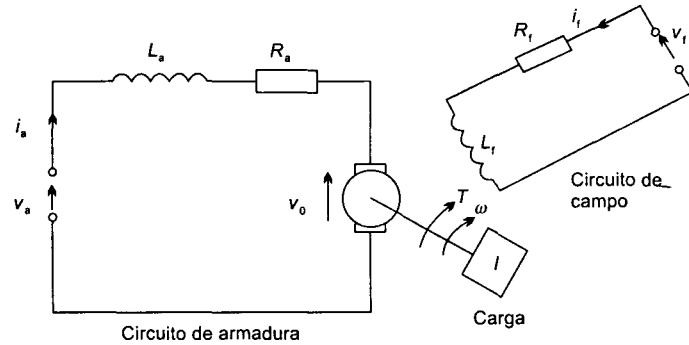
Figura 2.38 Circuitos del motor de cd
