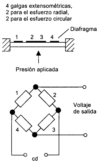
Figura 12.6 Celda de presión
