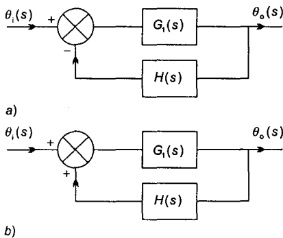
Figura 6.4 a) Realimentación negativa, b) realimentación positiva
