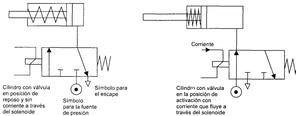
Figura 12.26 Control de un cilindro de acción simple
