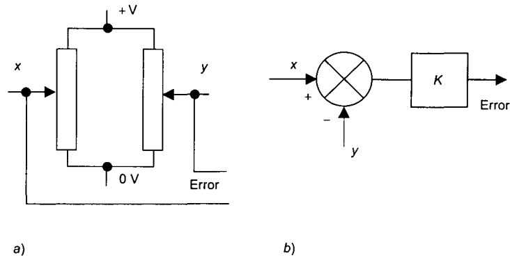
Figura 12.2 Sensor de error
