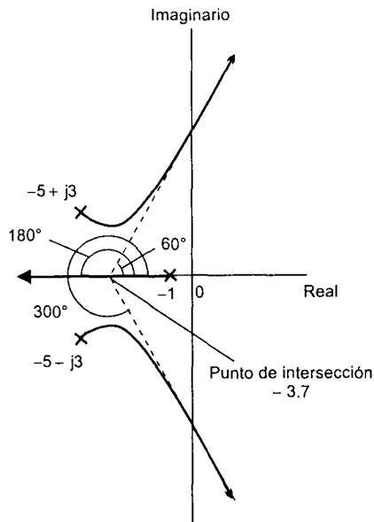
Figura 9.17 Asintotas con n = 3 y m = 0
