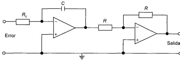
Figura 10.25 Controlador integral
