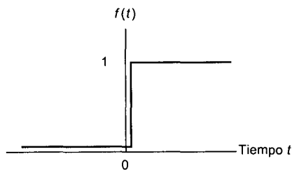
Figura 4.3 Una función escalón de altura 1
