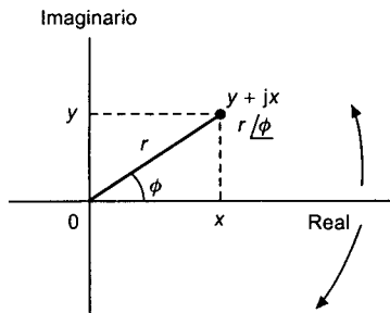
Figura 11.1 Un número complejo
