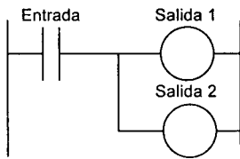
Figura 13.20 Salidas múltiples
