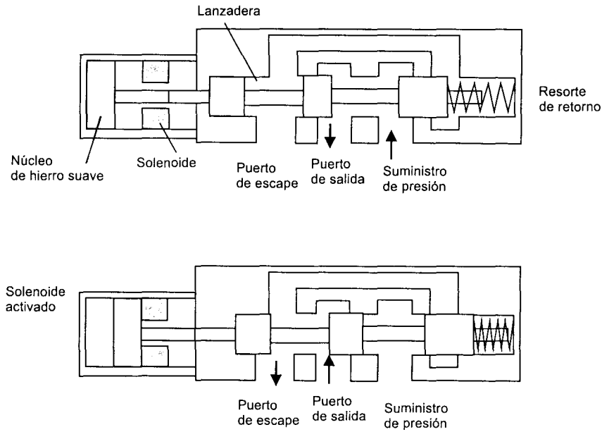
Figura 12.23 Válvula solenoide simple
