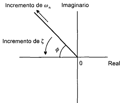
Figura 9.24 Frecuencia angular y factor de amortiguamiento relativo
