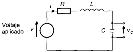
Figura 2.13 Sistema resistor-inductor-capacitor
