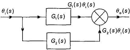
Figura 6.9 Lazo de prealimentación
