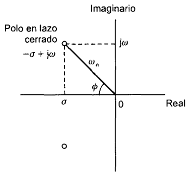
Figura 9.23 Polos complejos
