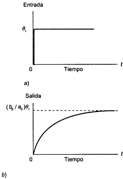
Figura 3.6 a) Entrada escalón para un sistema de primer orden y b) la salida resultante
