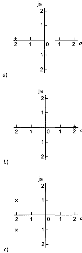
Figura 8.4 Patrones de polos y ceros y estabilidad, región de estabilidad compartida. a) Polo en -2 sin ceros: estable. b) Polo en +2 sin ceros: inestable. c) Polos en -2 \pm j1 sin ceros: estable.
