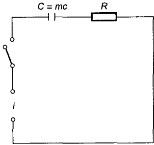
Figura 2.34 Analogía eléctrica de la figura 2.33
