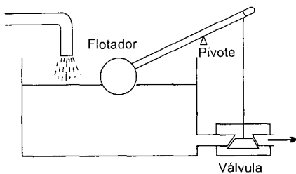
Figura 1.21 Sistema de control de nivel proporcional
