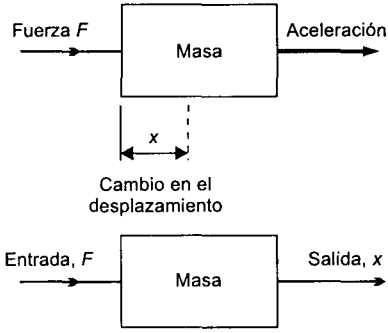
Figura 2.3 Un bloque funcional mecánico: la masa
