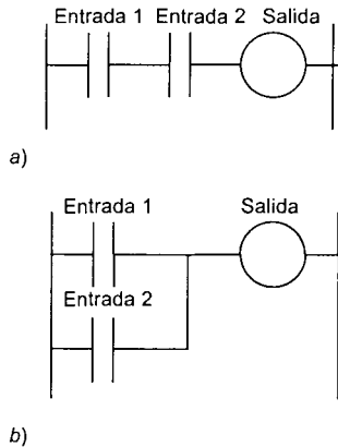
Figura 13.16 Compuertas lógicas: a) AND, b) OR
