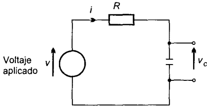
Figura 2.12 Sistema resistor-capacitor
