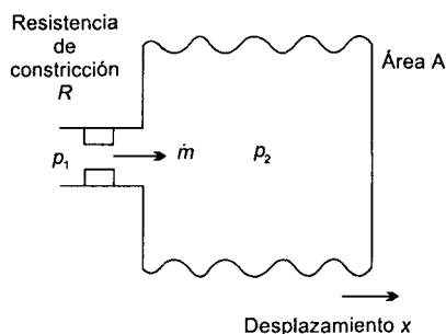
Figura 2.29 Un sistema neumático
