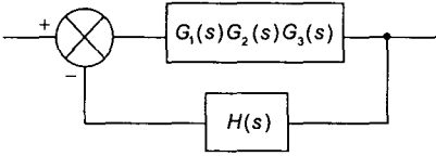
Figura 6.7 Sistema equivalente para la figura 6.6
