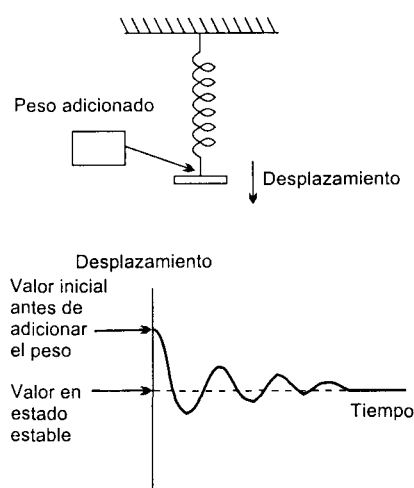
Figura 3.1 Respuestas transitoria y en estado estable de un sistema resorte
