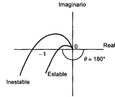
Figura 11.24 Trazas de Nyquist estable e inestable
