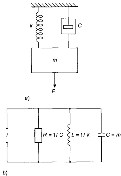
Figura 2.21 Analogías mecánica y eléctrica
