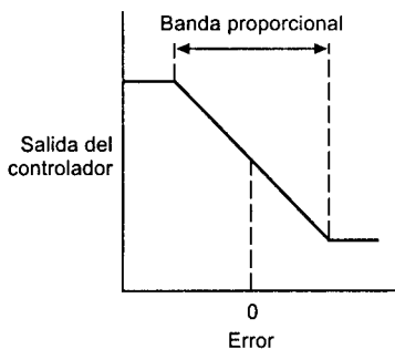
Figura 10.1 Control proporcional
