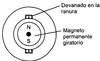
Figura 12.18 Motor de cd sin escobillas
