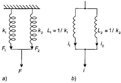
Figura 2.19 Analogías mecánica y eléctrica
