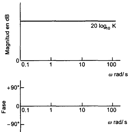
Figura 11.5 Trazas de Bode para una ganancia constante
