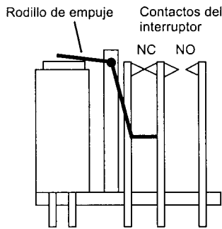
Figura 12.22 Relevador
