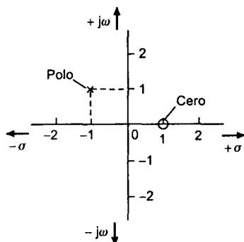
Figura 8.2 Patrón de polos y ceros
