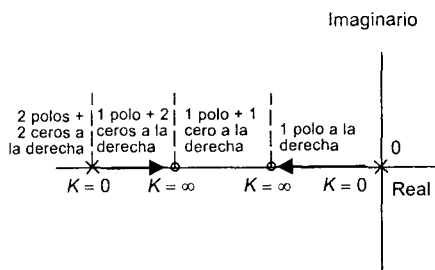
Figura 9.16 Lugares geométricos de las raíces sobre el eje real
