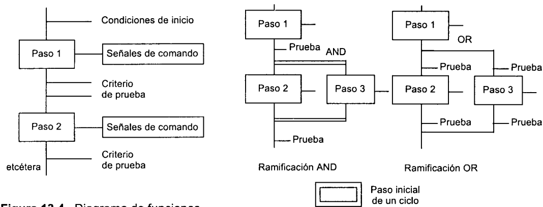
Figura 13.4 Diagrama de funciones
