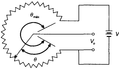
Figura 2.36 Potenciómetro
