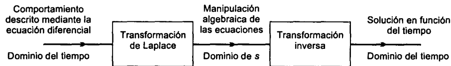
Figura 4.2 La transformación de Laplace
