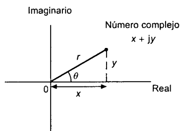
Figura 9.15 Figura polar de un número complejo
