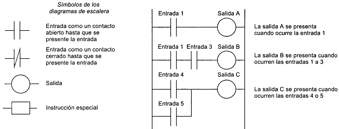
Figura 13.2 Diagrama de escalera
