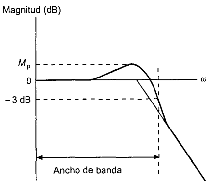
Figura 11.14 Especificaciones de desempeño
