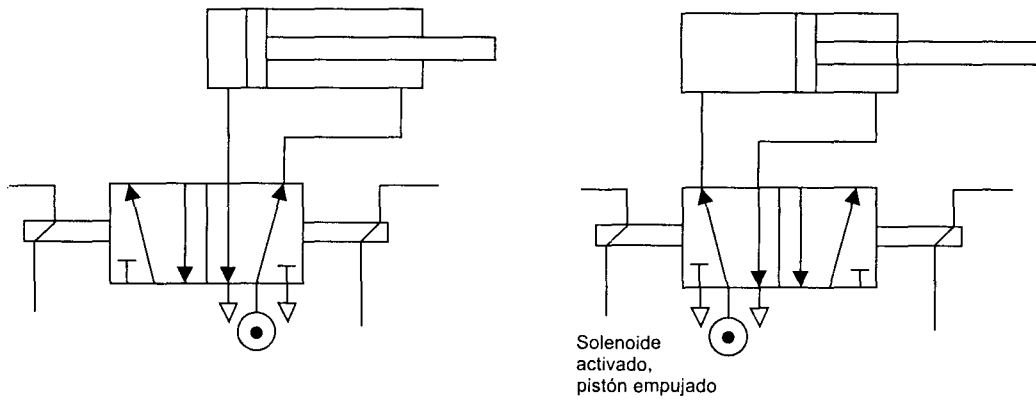
Figura 12.27 Control de un cilindro de doble acción
